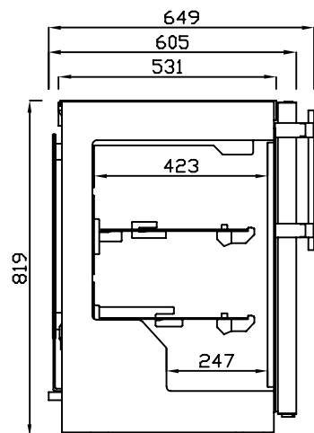
左側面図
