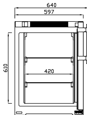
正面図 扉開放時
